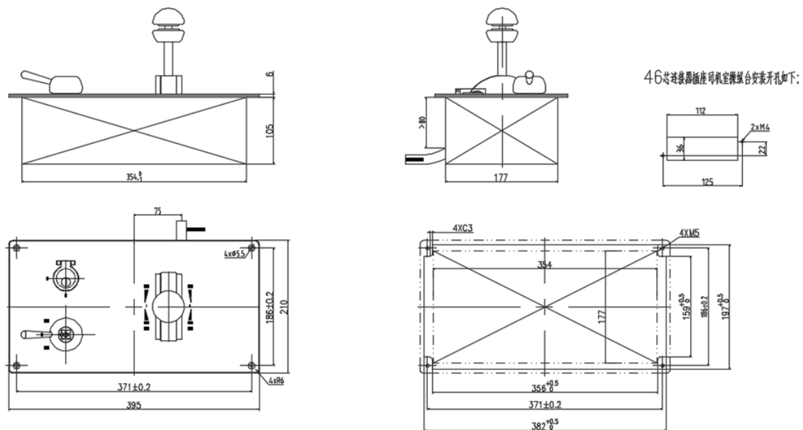
司机控制器外形及开孔图
